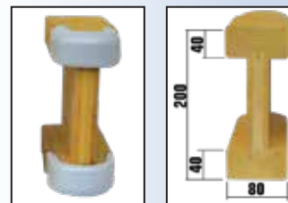
Embouts avec renforts
